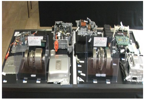
動力分割機構の比較
