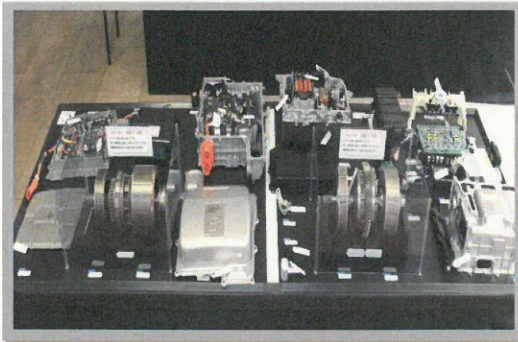
2代目プリウス・HV制御部品(左)と3代目プリウス・HV制御部品
